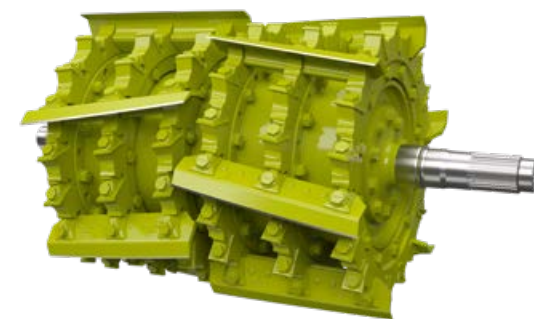
Trešdaļa no pilnas nažu sekcijas (ar V36), lai palielinātu smalcināšanas garumu ar simetrisku augu masas padevi.
