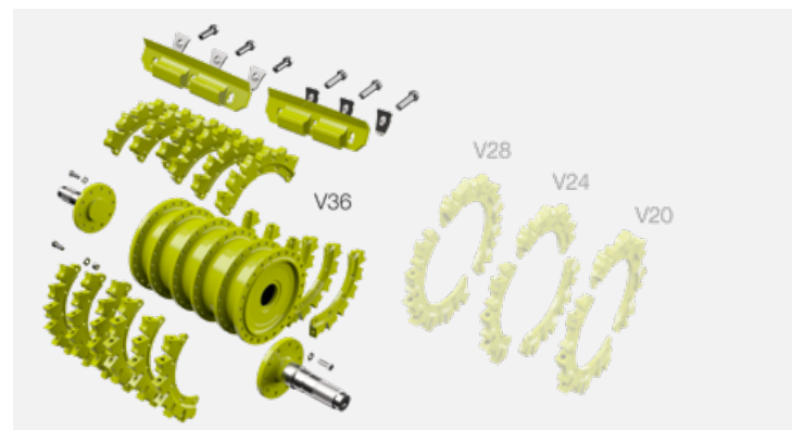
Smalcinātāja rotoru korpusu var aprīkot ar 36, 28, 24 vai 20 nažiem.
