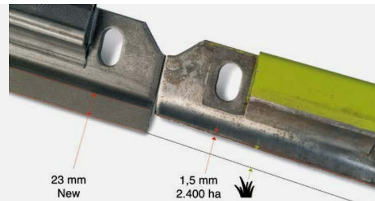
V-FLEX nažiem ir 23 mm biezs pretnodiluma pārklājums.
