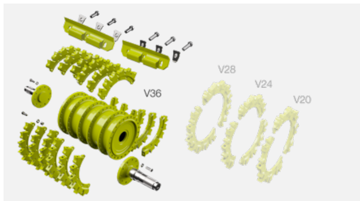
Ant smulkinimo būgno korpuso galima sumontuoti 36, 28, 24 arba 20 peilių.
