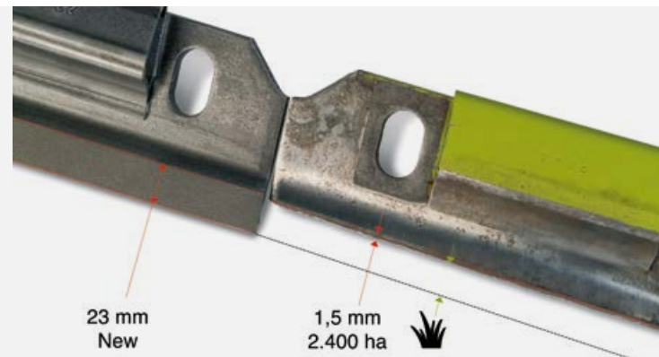
V-FLEX peilių dilimui atspari danga yra 23 mm pločio.
