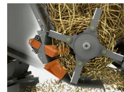
Protioštrí a výkyvný prvek dna řezačky slámy v SPECIAL CUT.
