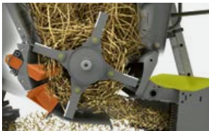
Broyeur SPECIAL CUT avec contre-couteau et fond rotor à élément escamotable
